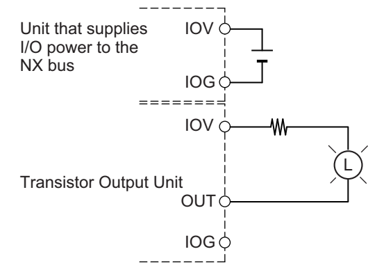
NPN type
