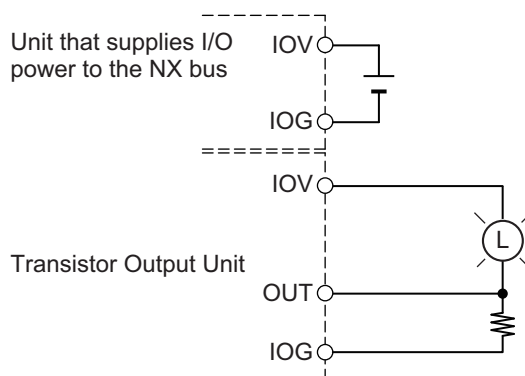
NPN type
